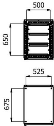
W-W ( 1 : 30 )
