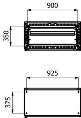
U-U ( 1 : 25 )
