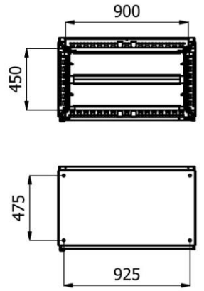
N-N ( 1 : 25 )
