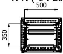
N-N ( 1 : 20 )
