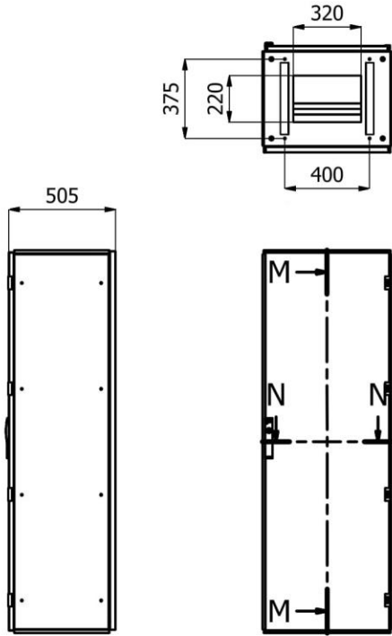
N-N ( 1 : 20 )
