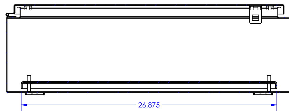
SECTION D-D
