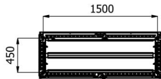
U-U ( 1 : 30 )
