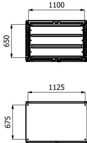
U-U ( 1 : 30 )
