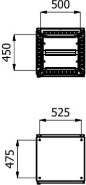
W-W ( 1 : 30 )
