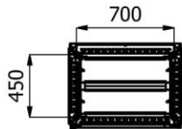
N-N ( 1 : 30 )
